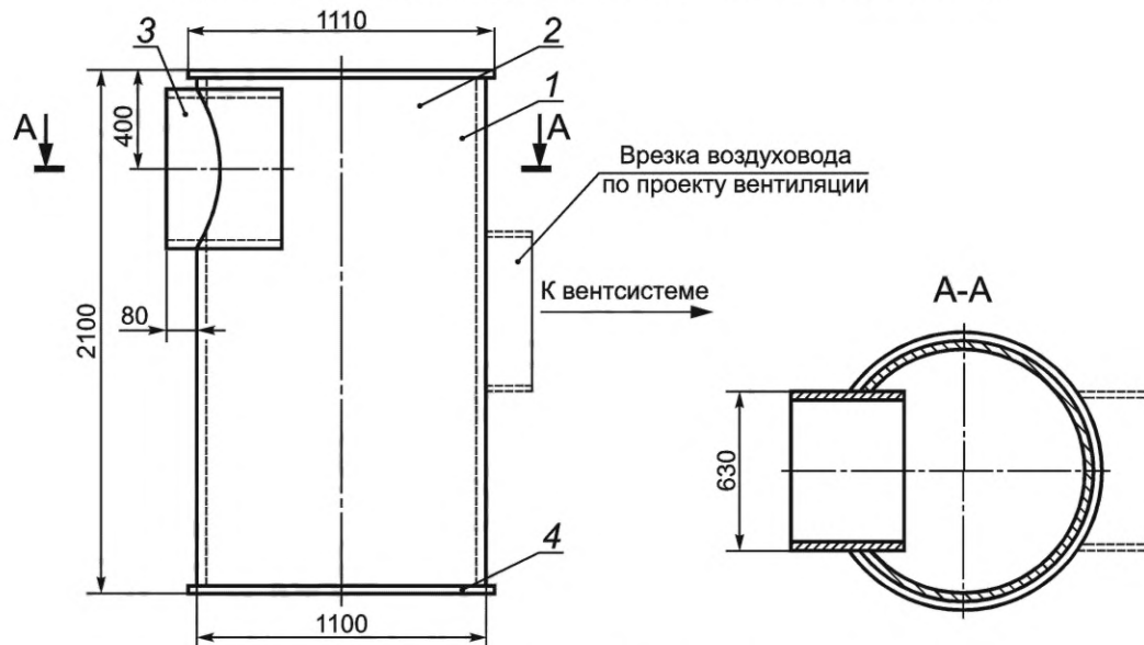
Рисунок А.1 — Схема конструктивного исполнения РК объемом 0,5 м³
