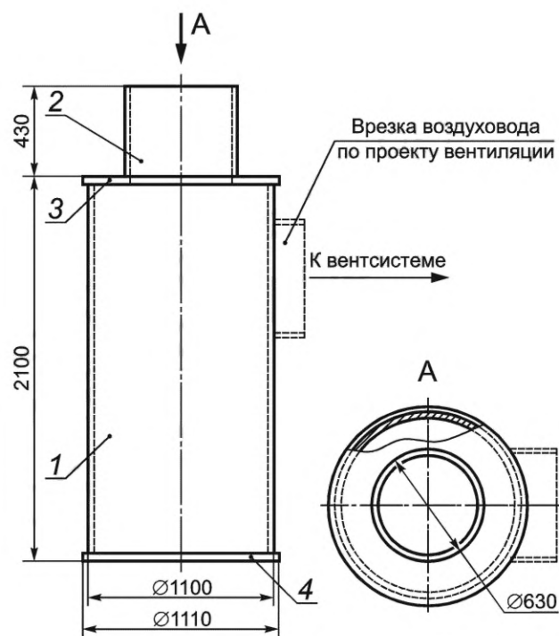
Рисунок А.3 — Схема конструктивного исполнения РК объемом 2,0 м 3 при присоединении воздухопроводов сверху
