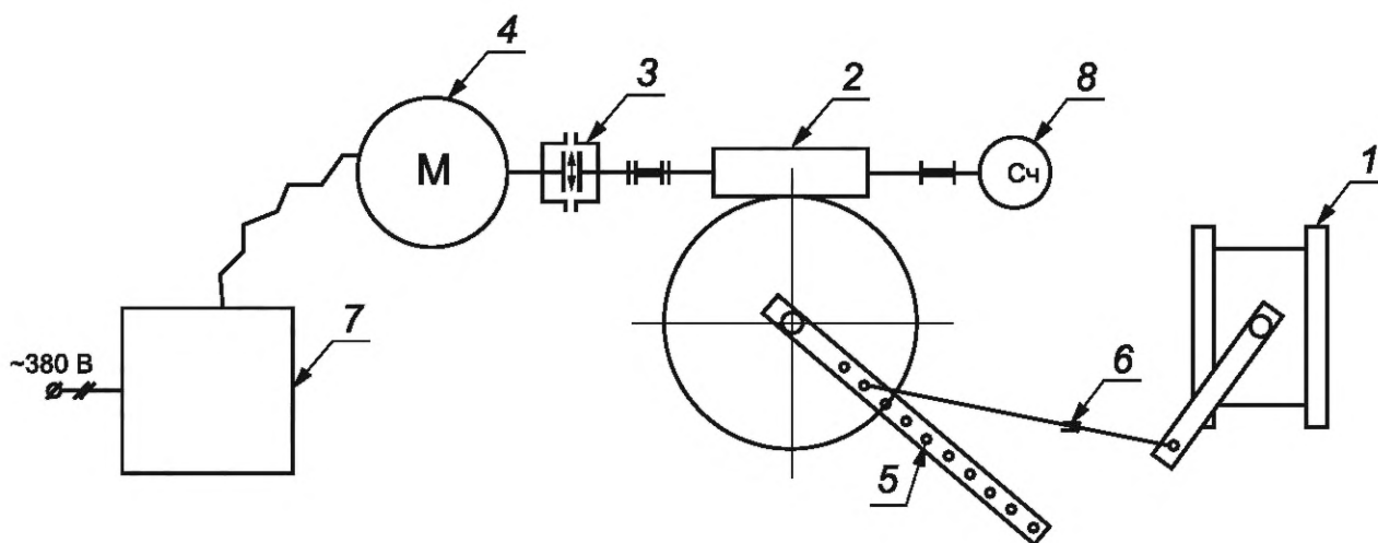
Рисунок Б.5 — Принципиальная схема станда для определения коэффициента сопротивления герметических клапанов
