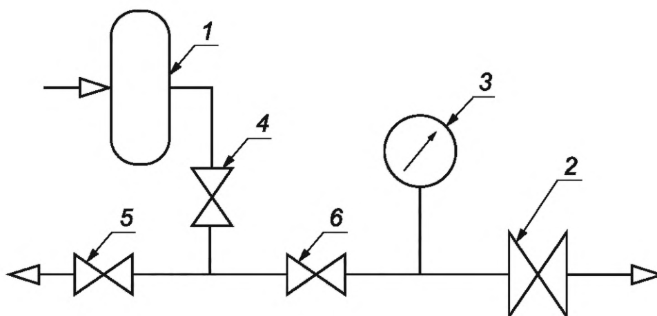
Рисунок Б.4 — Рекомендуемая схема стенда для испытания ГК на герметичность затворов клапанов манометрическим методом
