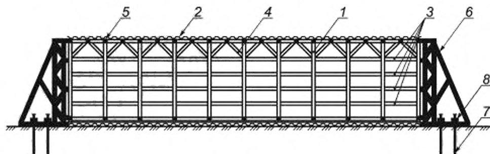
1 — вертикальные стойки; 2 — наружный профлист; 3 — горизонтальные балки; 4 — наклонные балки; 5 — поперечные балки; 6 — контрфорсы; 7 — анкера; 8 — гайки
