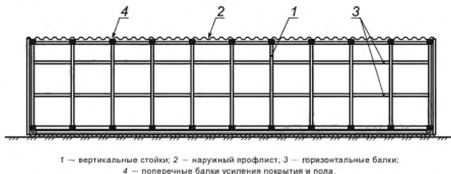
Рисунок 9 — Пример продольного разреза базового блок-модуля Укр ГО БМТ с элементами усиления
