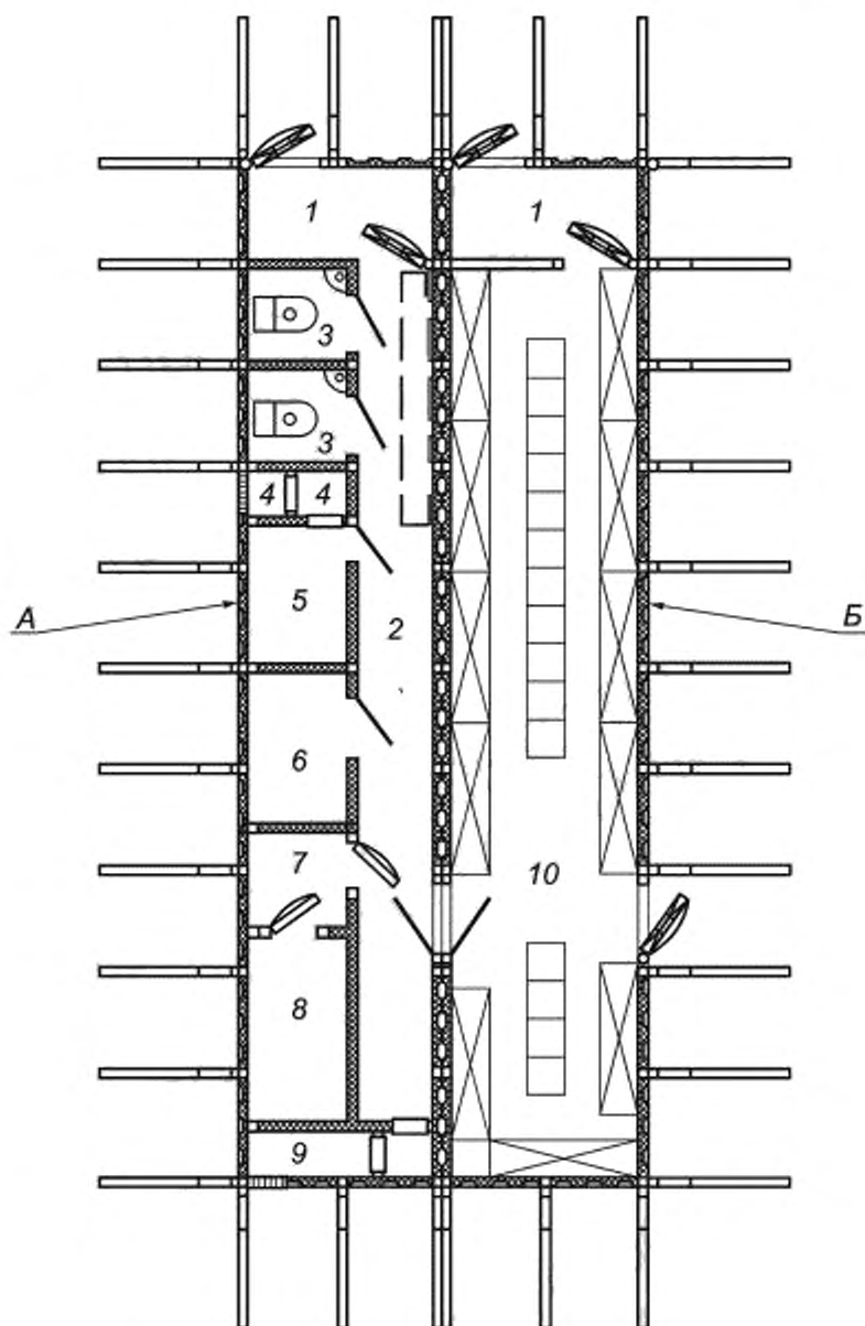
А — технический блок-модуль; Б — блок-модуль для размещения укрываемых. 1 — входной тамбур-шлюз; 2 — коридор; 3 — туалет; 4 — расширительная камера; 5 — ФВК; 6 — помещение для баллонов с воздухом; 7 — тамбур ДЭС; 8 — ДЭС; 9 — расширительная камера для охлаждения ДГ; 10 — помещение для укрываемых
