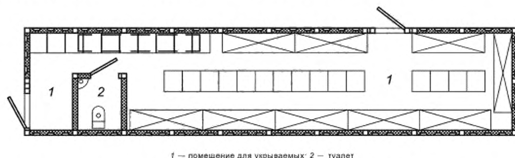
Рисунок 10 — Пример объемно-планировочного решения Укр ГО БМТ ПРУ
