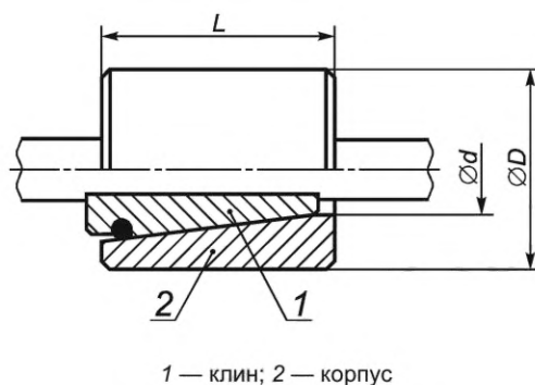
Рисунок 1 — Открытый зажим
