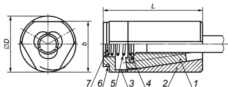
Рисунок 3 — Закрытый зажим. Исполнение 2
