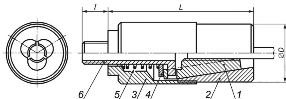
Рисунок 2 — Закрытый зажим. Исполнение 1
