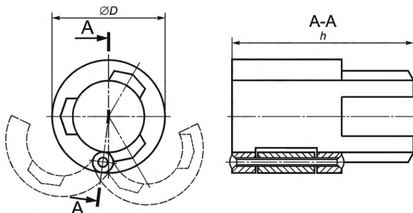
Рисунок 9 — Шарнирная вилка для съема закрытого зажима исполнения 2
