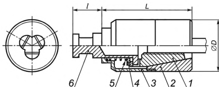
Рисунок 4 — Закрытый зажим. Исполнение 3
