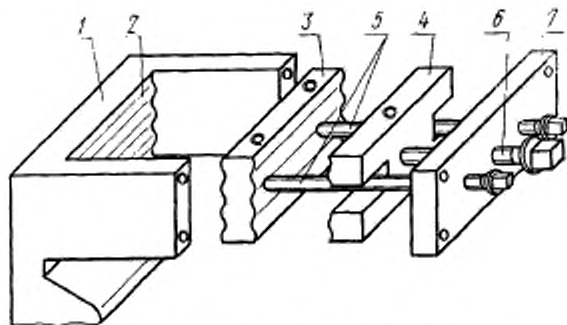
1—корпус зажима; 2—неподвижная губка; 3—промежуточная подвижная губка; 4—крайняя подвижная губка; 5—зажимные болты; 6—прижимной винт; 7—прижимная планка.
