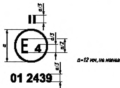
Схема знака официального утверждения зеркала заднего вида (см. 5.4 настоящих Правил)
