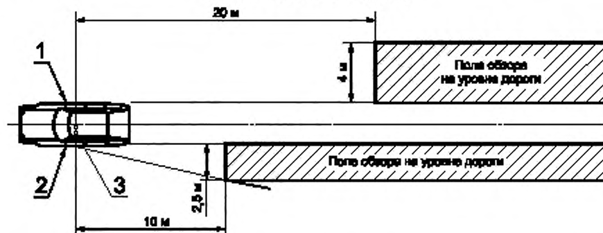
1 — правое внешнее зеркало заднего вида; 2 — левое внешнее зеркало заднего вида; 3 — окулярные точки водителя
