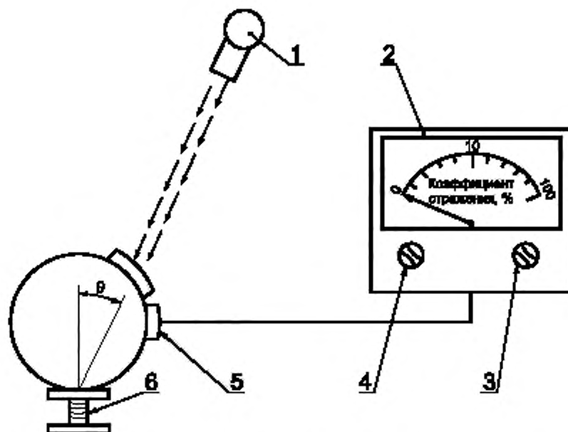
1 — источник света и коллиматор; 2 — регулируемый индикатор; 3 — регулировка градуирования; 4 — установка на ноль; 5 — фотоземлет; 6 — штатив для закрепления образца
