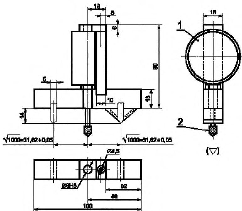
1 — компаратор; 2 — подвижная точка
