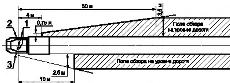
1 — окулярные точки водителя; 2 — правое внешнее зеркало заднего вида; 3 — левое внешнее зеркало заднего вида
