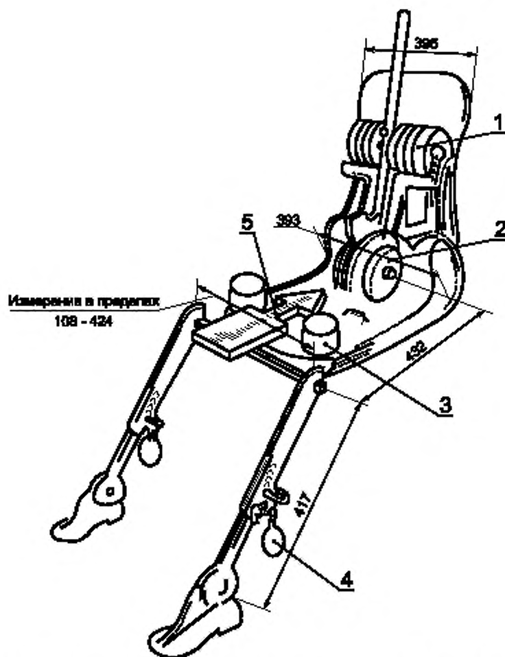
1 — спинные грузы; 2 — сидельные грузы; 3 — набедеренные грузы; 4 — ножные грузы; 5 — направление и точка приложения нагрузки
