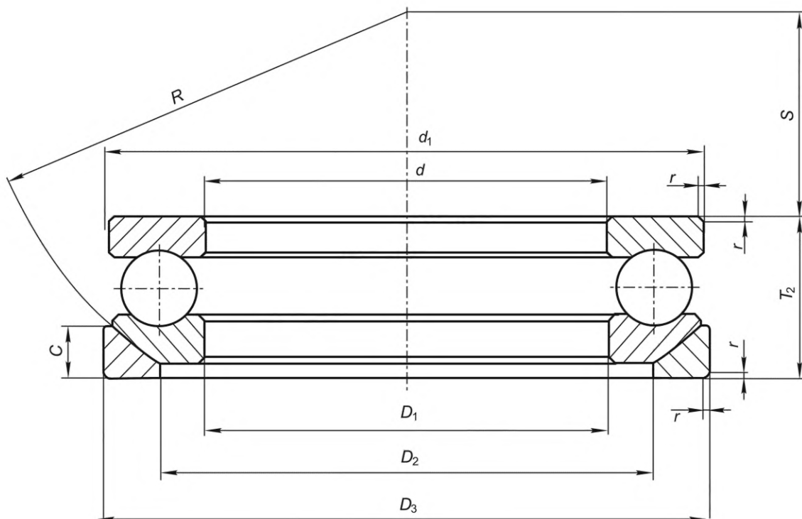
Рисунок 2 — Конструктивное исполнение 01
