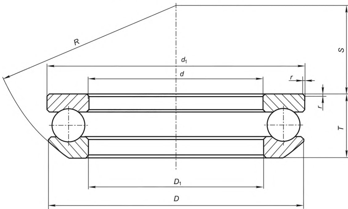
Рисунок 3 — Конструктивное исполнение 02
