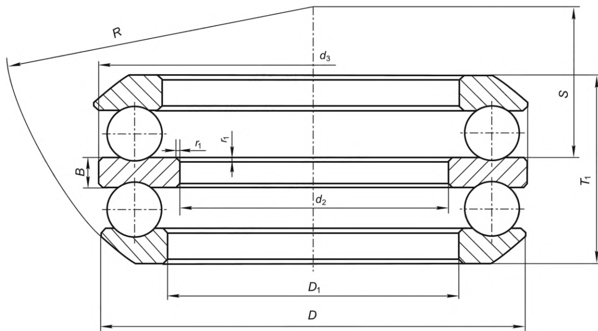
Рисунок 6 — Конструктивное исполнение 05
