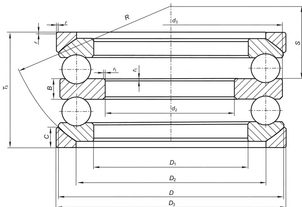
Рисунок 5 — Конструктивное исполнение 04
