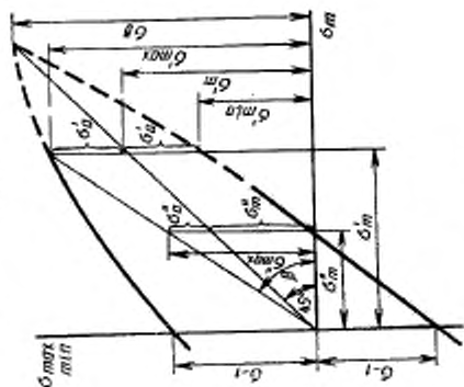
Диаграмма предельных напряжений цикла
