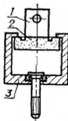
1—испытательная головка; 2—образец; 3—захват.
