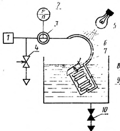
Схема установки для испытания фильтрующе-поглощающих коробок противогазов
