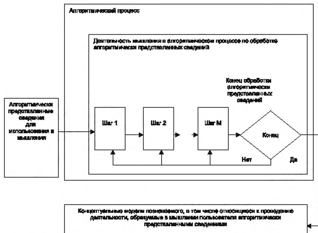
Рисунок 3 — Алгоритмический процесс в мышлении пользователя при проведении им деятельности с использованием алгоритмически представленных сведений
