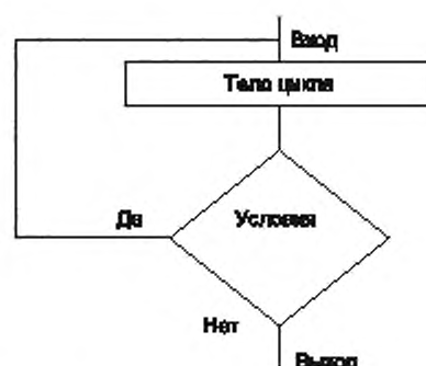
Рисунок 7 — Информационная структура «цикл-до»
