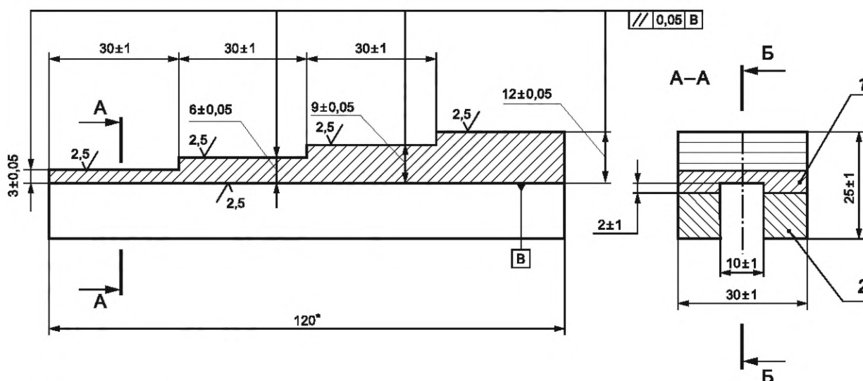
Рисунок 8 — НО типа ТН2 для настройки дефектоскопа при измерении толщины АНП со стороны наплавленной поверхности
