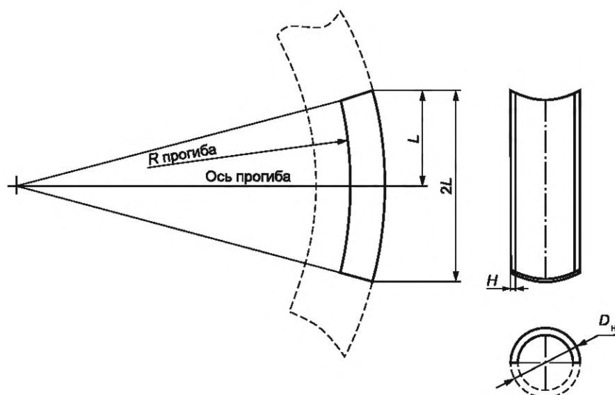
Рисунок 12 — НО в виде участкагиба (колена) трубопровода
