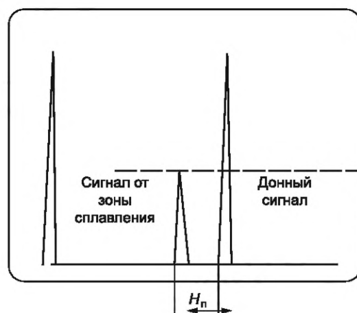
Рисунок 22 — Измерение толщины АНП с применением НП
