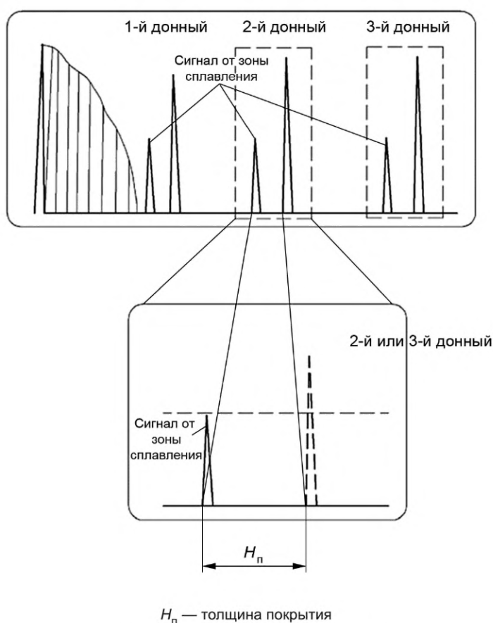
Рисунок 21 — Экран дефектоскопа при измерении толщины АНП на биметаллической трубе и с увеличенным масштабом развертки
