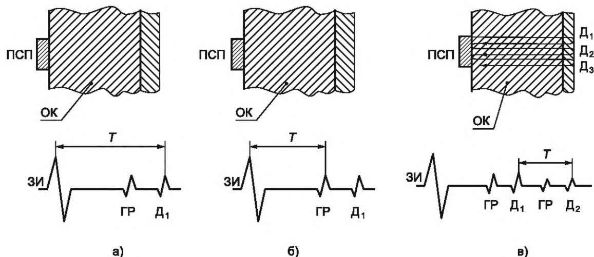
Рисунок 2 — Способы измерения толщины биметалла
