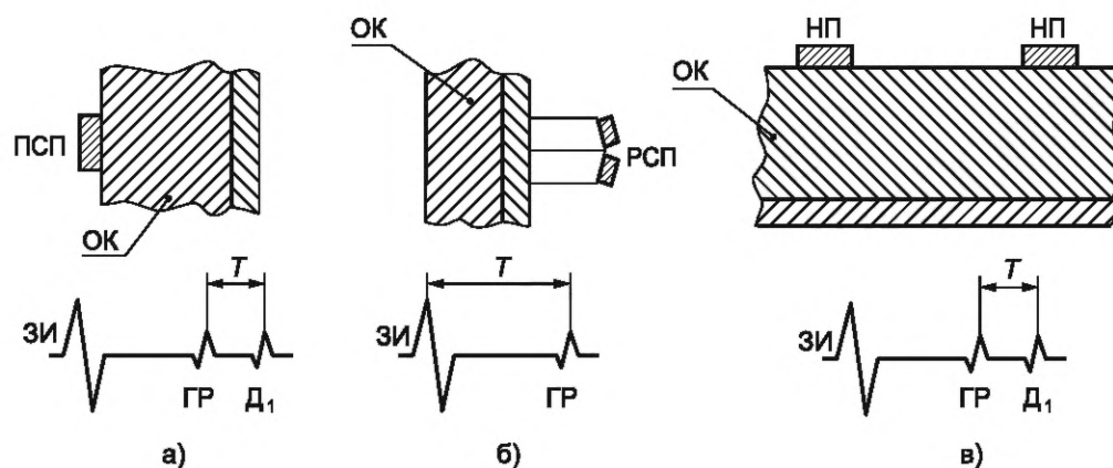
Рисунок 3 — Способы измерения толщины АНП
