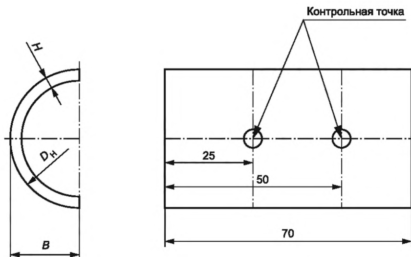
Рисунок 11 — НО в виде участка трубы
