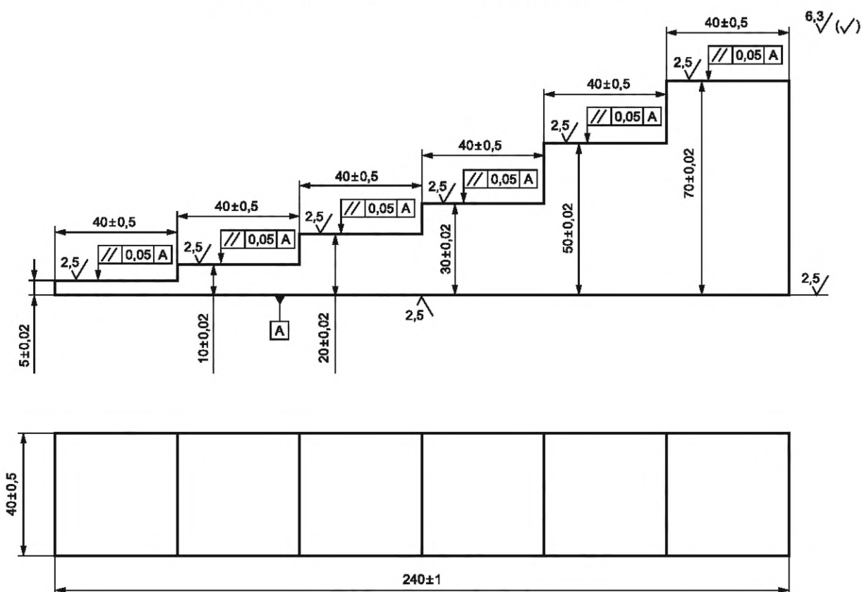
Рисунок 13 — НО типа НОТ-1
