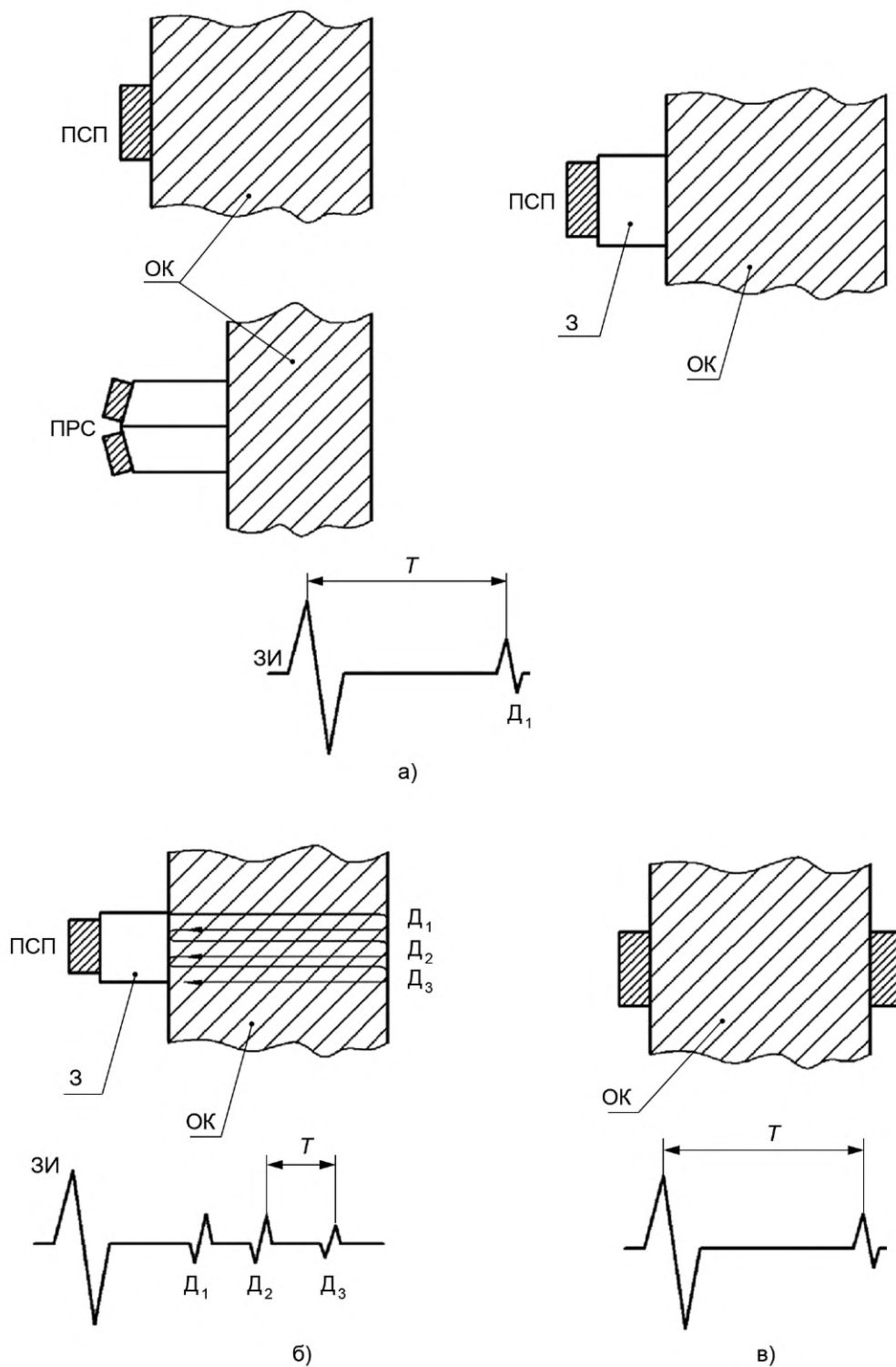
Рисунок 1 — Способы измерения толщины монометалла
