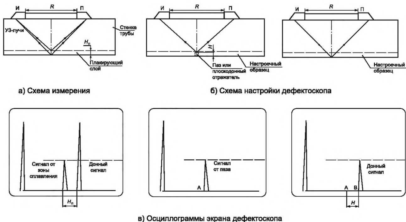
Рисунок 17 — Настройка параметров дефектоскопа при измерении АНП с применением НП на образце ТНН1
