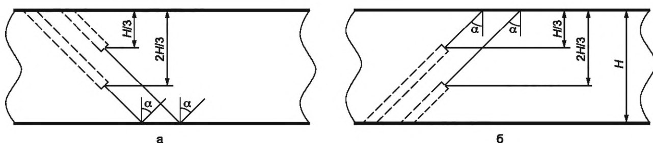
Рисунок 7 — Пример расположения ПДО для УЗК АСС с номинальной толщиной сварной детали свыше 10 до 20 мм
