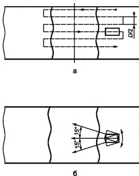
а — сканирование на продольные несплошности; б — поворот ПЭП при сканировании; D — диаметр (ширина) пьезоэлемента
