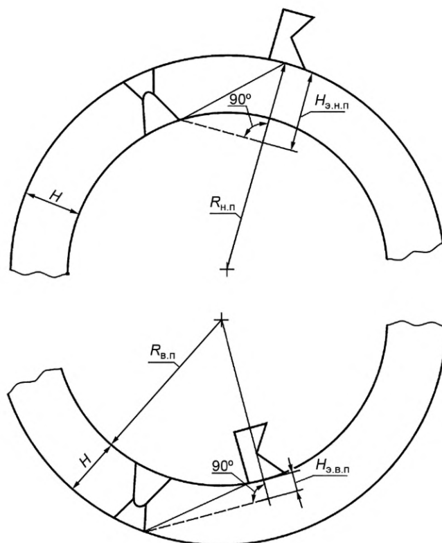
Рисунок В.1 — Эквивалентные плоскому АСС толщины H_{э.н.п} и H_{э.в.п} АСС оборудования цилиндрической формы
