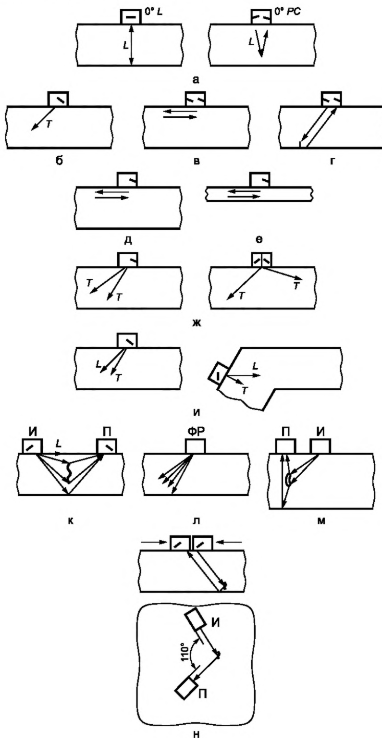
Рисунок 1 — Операции прозвучивания
