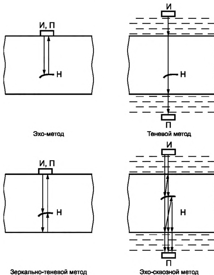
Рисунок 2 — Методы УЗК продольными волнами
