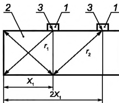
1 — ПЭП; 2 — изделие; 3 — точка ввода
