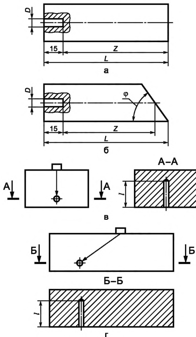
Рисунок 5 — Настроечные образцы
