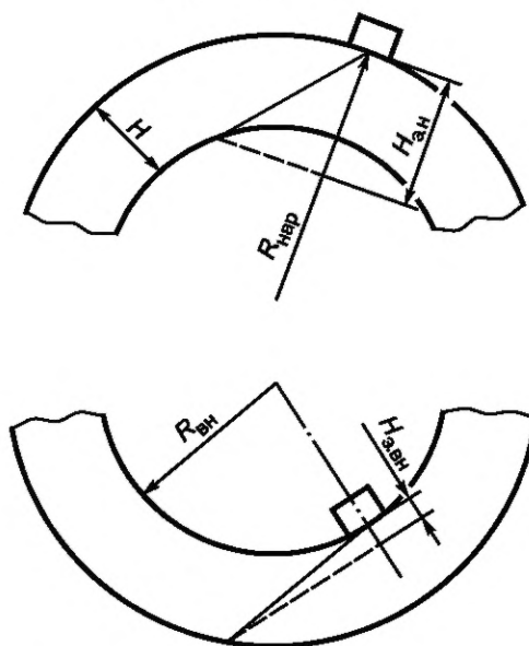
Рисунок 6 — Эквивалентная толщина ОК цилиндрической формы
