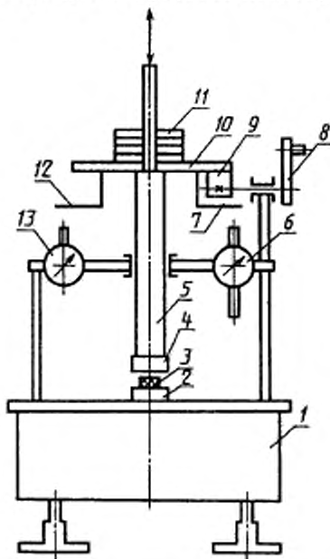
Схема прибора для определения хладотекучести
