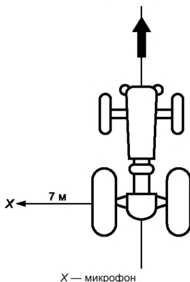
Рисунок 2 — Схема измерений внешнего шума неподвижного трактора
