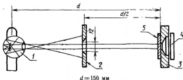
1 — проекционная лампа; 2 — промежуточная маска; 3 — измерительная маска; 4 — фотозлемент; 5 — дюза
