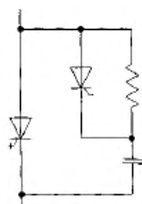
Рисунок A.1d — Пример гасящего контура
