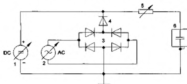
Рисунок 2 — Источник постоянного тока N — Тип 1
