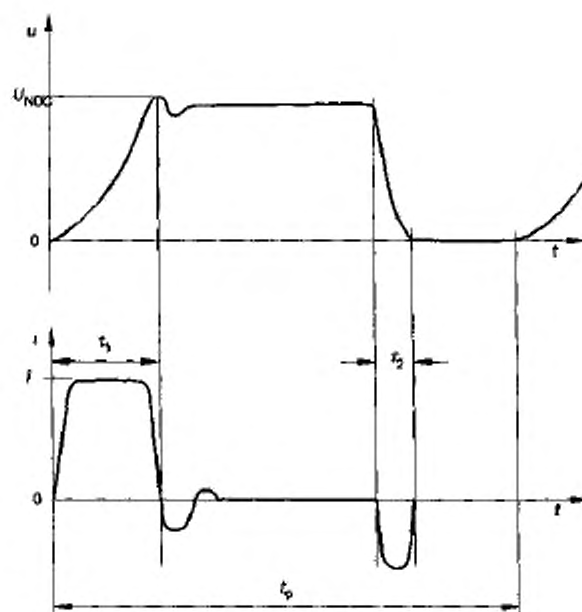
Рисунок A.1c — Форма сигнала для гасящих конденсаторов для запираемых тиристоров
