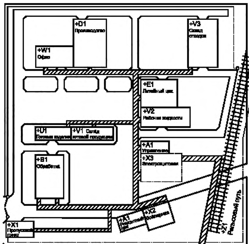
Рисунок 87 — Компановочный чертеж промышленного предприятия
