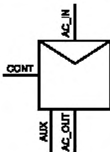
Рисунок 97 — Символ пускателя электродвигателя, предназначенный для использования в однолинейных представлениях
