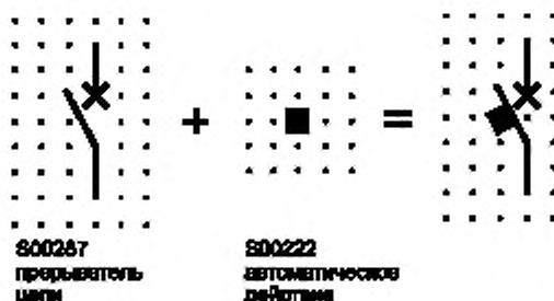
Рисунок A.4 — Микровыключатель, показанный как комбинация символа прерывателя цепи и спецификатора, подчеркивающего автоматическое срабатывание
