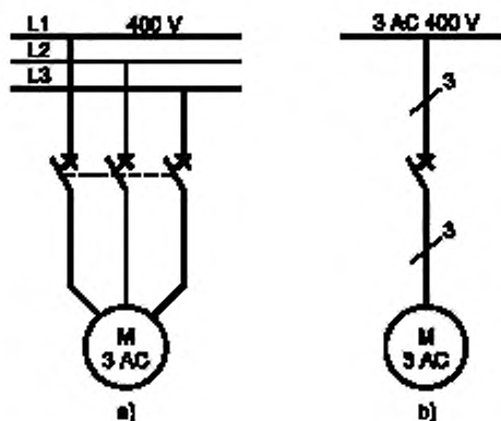
Рисунок 53 — Пример представления многофазной цепи
