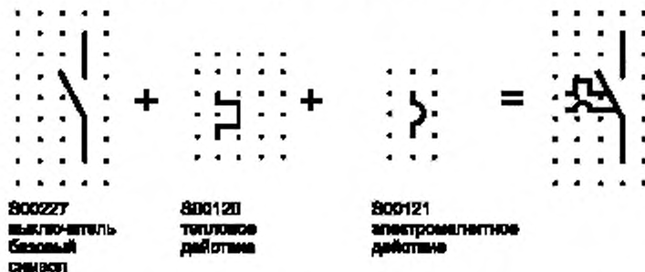
Рисунок A.5 — Микровыключатель, показанный как комбинация символа выключателя и спецификаторов, подчеркивающих тепловой и электромагнитный эффекты
