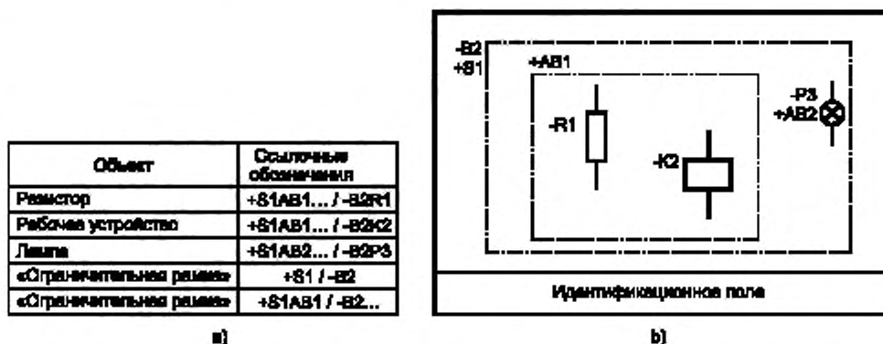
Рисунок 46 — Представление групп ссылочных обозначений в ограничительной рамке
