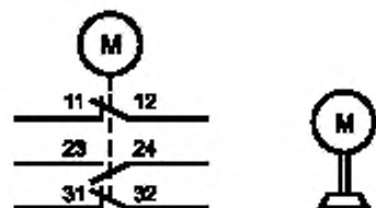
Рисунок 32 — Пример представления механических связей
