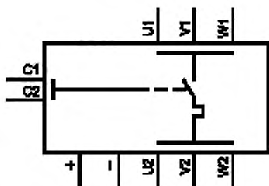
Рисунок 95 — Символ пускателя электродвигателя
