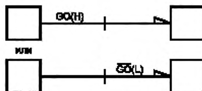
Рисунок 76 — Примеры указателей несовпадения полярности
