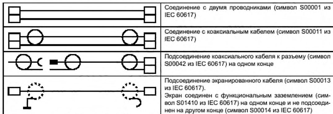
Рисунок 80, лист 1 — Пример кабельных соединений
