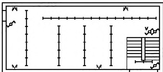
c) Базовый чертеж с добавлением устанавливаемых светильников
