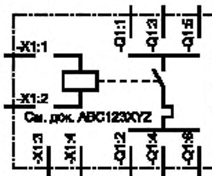
Рисунок 94 — Пример схемного представления пускателя двигателя
