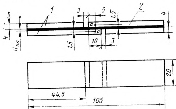
1—металл; 2—клеевой слой; ас—база измерения деформации
