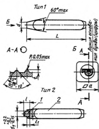
1 — вставка; 2 — державка
