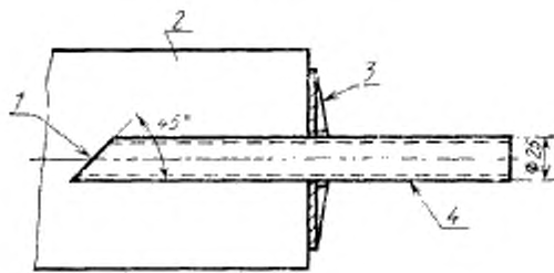
1 — центр мешка; 2 — мешок; 3 — горловина мешка; 4 — трубка
