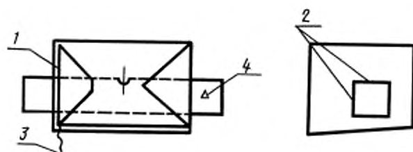
1 — прорезь; 2 — опорные плоскости; 3 — нитка; 4 — метка
