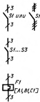
б — однолинейное изображение
