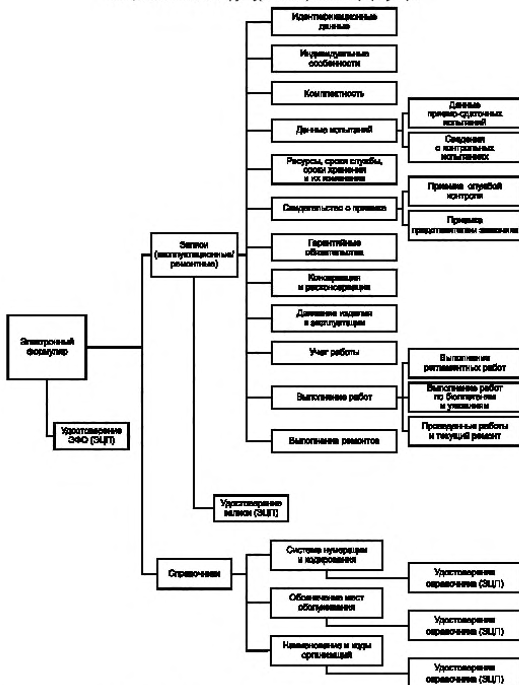
Рисунок Б.1 — Логическая структура электронного формуляра
