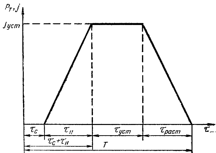
Схема тормозной диаграммы
