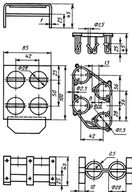
Подставка для тиглей
