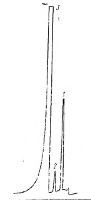
1—изопропиловый спирт; 2—этиловый спирт; 3—метанол
