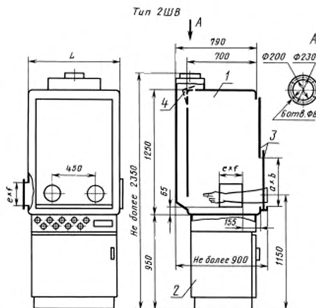
1 – корпус; 2 – опора; 3 – шторки; 4 – регулирующая заслонка
