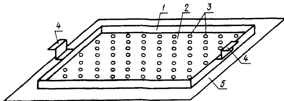
1—прямоугольная коробка; 2—дно с отверстиями; 3—отверстия круглой формы; 4—ручки; 5—плоская подставка
