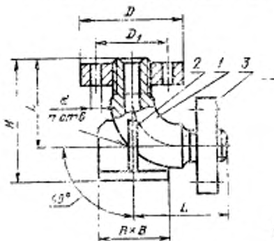
1 — колено по ГОСТ 22794—83; 2 — опора по ГОСТ 22797—83; 3 — фланец по ГОСТ 9399—81
