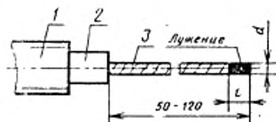
1—баллон; 2—токовый вывод; 3—гибкий вывод
