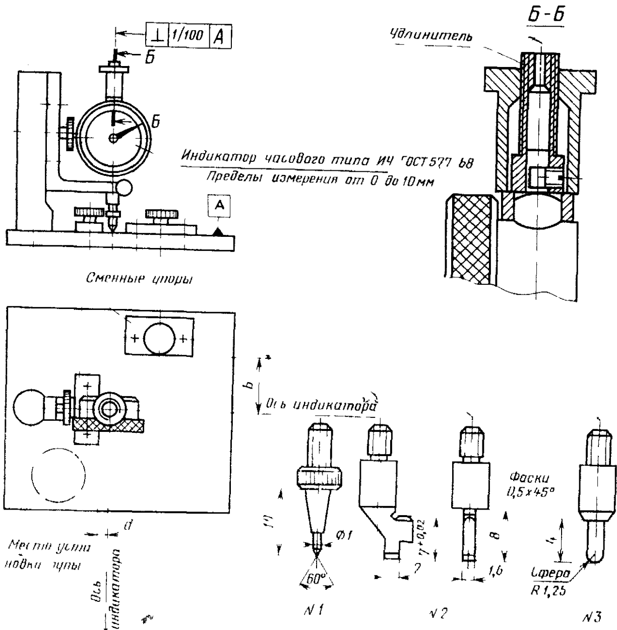
Индикаторное приспособление
