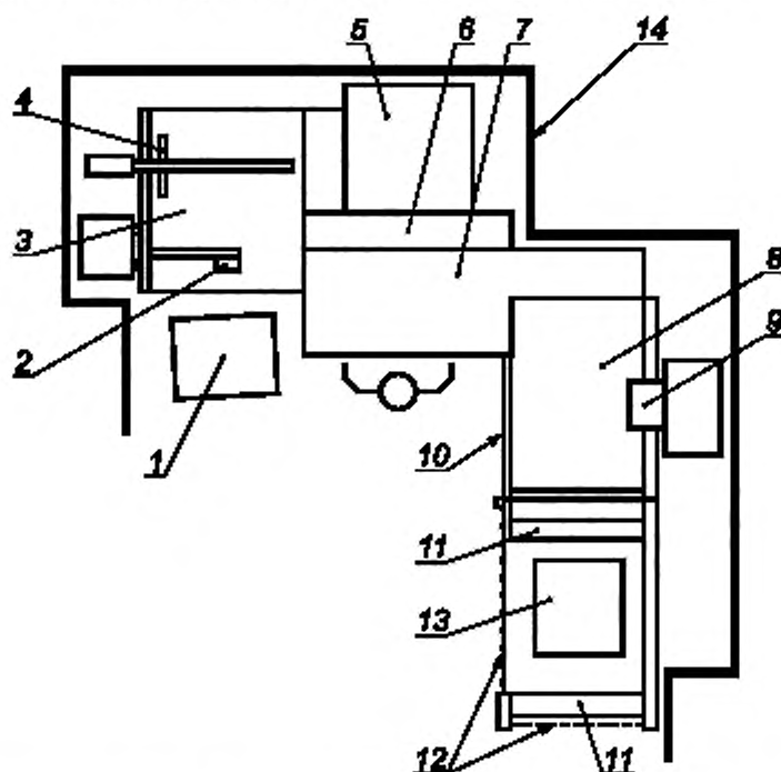
1 — бумажный стель; 2 — щипцовый захват; 3 — загрузочный стол; 4 — толкатель; 5 — задний стол; 6 — машина резальная; 7 — передний стол; 8 — разгрузочный стол; 9 — прижим; 10 — ограждение; 11 — приемный упор; 12 — ЭЧПУ; 13 — поддон; 14 — ограждение
