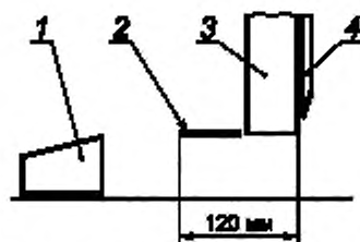
1 — затл; 2 — ограждение; 3 — балка прижима; 4 — нож
