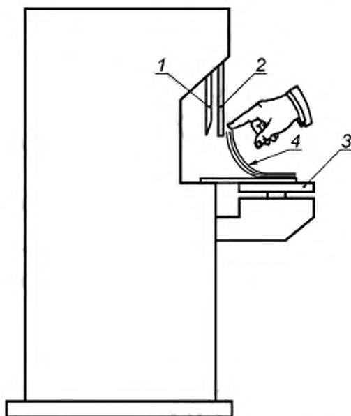
1 — нож; 2 — опережающее ограждение (отрагатель); 3 — накладной стол; 4 — книжный блок
