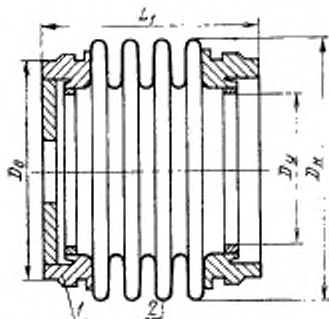
1—присоединительный сильфон; 2—патрубок; Черт. 5
