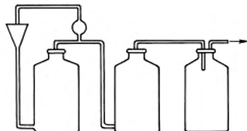
Установка для удаления ртути из сточных растворов
