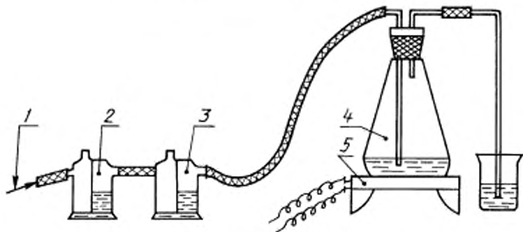
1 — углекислый газ; 2 — промывная склянка с раствором меди (50 г/дм 3 ); 3 — промывная склянка с водой; 4 — коническая колба (5.1); 5 — плита для нагревания
