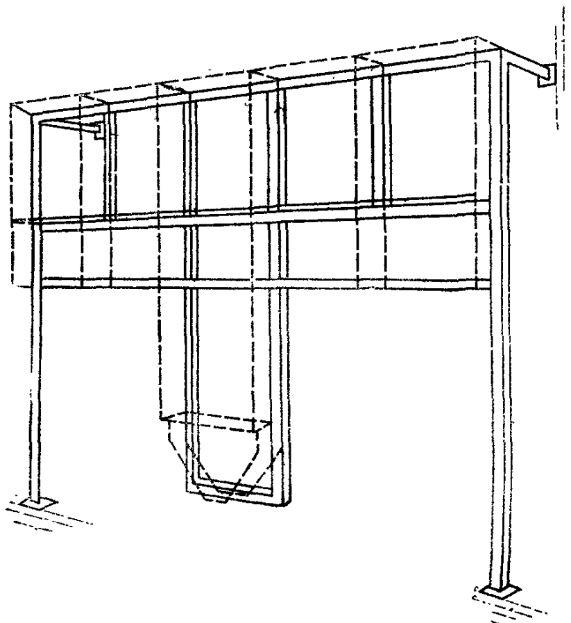
Рисунок С.8 — Монтажная конструкция
