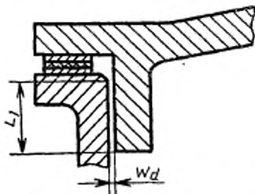
Цилиндрическое взрывонепроницаемое соединение с металлопластической прокладкой для оболочек подгруппы ИС
