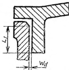
Цилиндрическое взрывонепроницаемое соединение для оболочек подгруппы ИС
