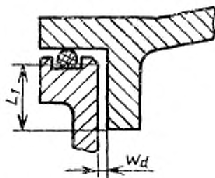
Цилиндрическое взрывонепроницаемое соединение с эластичкой прокладкой для оболочек подгруппы ИС
