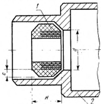
1 — уплотнительное кольцо для кабеля; 2 — корпус кабельного ввода; d — диаметр проходного отверстия; H — высота уплот- нительного кольца; \delta — толщина уплотни- тельного кольца
