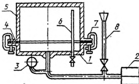
1 — стенд для гидрокиспытаний; 2 — устройство для создания давления воды (насос); 3 — прибор для измерения давления; 4 — резиновая прокладка; 5 — испытываемая деталь; 6 — трубка для выхода воздуха при заполнении водой; 7 — трубка для крепления испытываемой детали к стенду; 8 — трубка для предварительного заполнения оболочки водой
