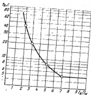
График определения минимального значения времени нагрева t_e
