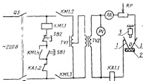
Принципиальная электрическая схема установки испытаний на трекингостойкость
