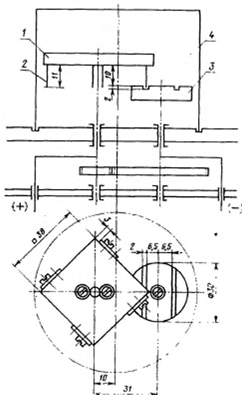
1—диск для крепления подвижных контактов; 2—вольфрамовая проволока; 3—клиновидный диск; 4—вырванная камера
