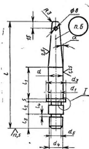
Штыри центрирующие
