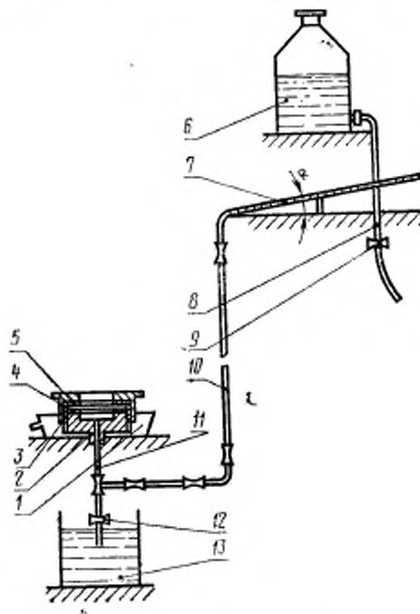
1—ванна; 2—полую камера; 3—крышка; 4—резиновая уплотняющая прокладка; 5—металлическая прокладка; 6—сосуд с тубусом для воды; 7—стеклянная градуированная трубка; 8, 11—резиновые трубки; 9, 12—зажимы на трубках; 10—стеклянная трубка; 13—бачок для сбора воды.
