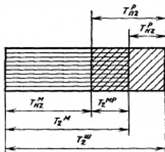
Хронограмма второго состояния
