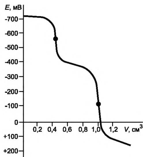
Рисунок А.3 — Кривая потенциометрического титрования сульфид- и меркаптитд-ионов раствором азотнокислого аммиаката серебра
