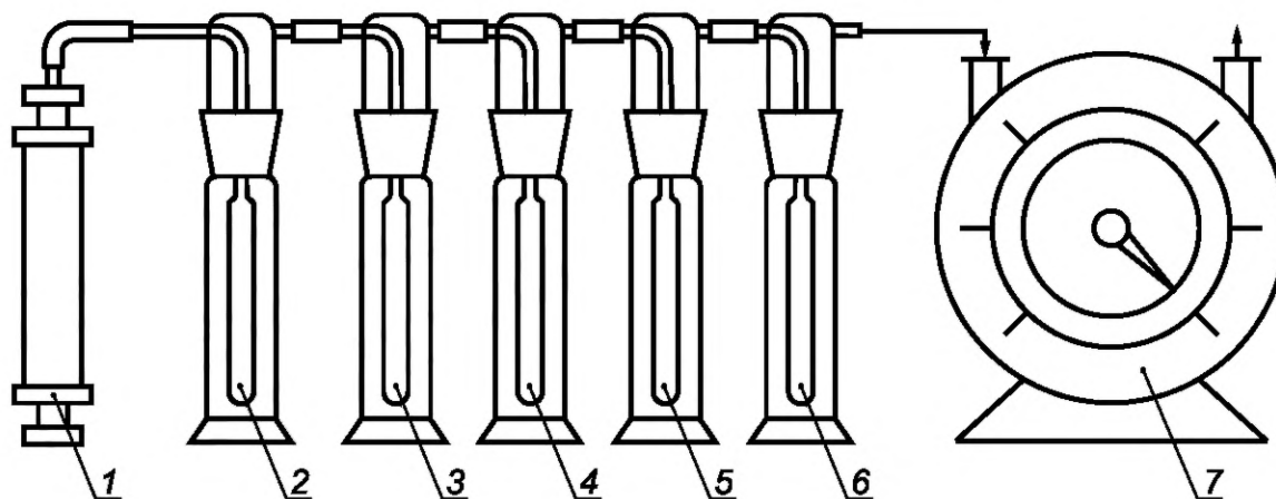
1 — прободоотборник; 2 — предохранительная склянка; 3—6 — поглотительные склянки; 7 — газовый счетчик
