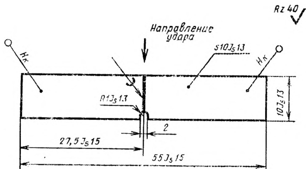
Черт. 2
