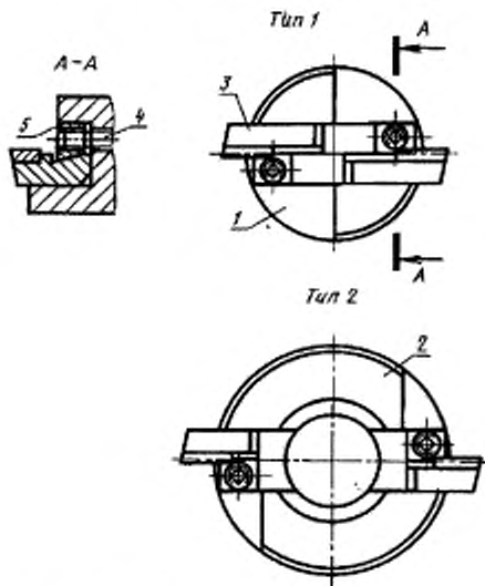
Головки типов 1 и 2 (черт. 1)
