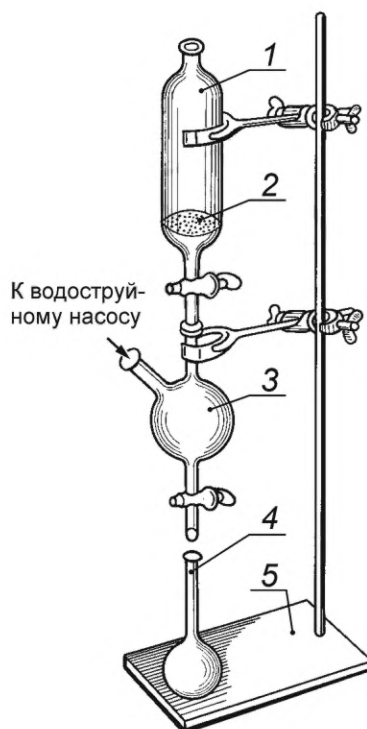
1 — фильтрующая делительная воронка; 2 — впаянный стеклянный фильтр класса ПОР 100 или ПОР 160; 3 — приемник; 4 — мерная колба; 5 — штатив
