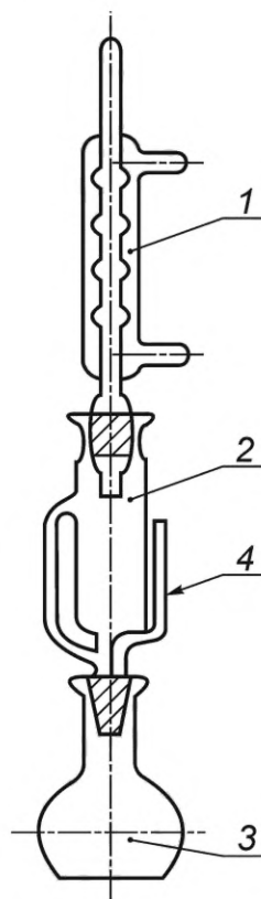
1 — холодильник; 2 — экстрактор; 3 — экстракционная колба; 4 — сифонная трубка
