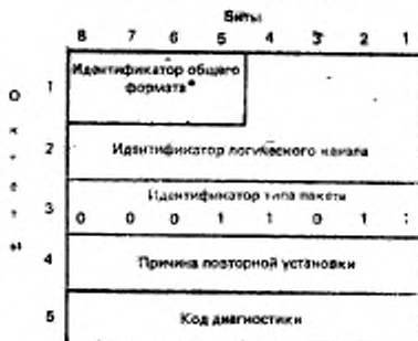
Черт. 19 Формат пакета ЗАПРОС ПОВТОРНОЙ УСТАНОВКИ и ИНДИКАЦИЯ ПОВТОРНОЙ УСТАНОВКИ
