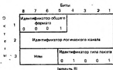
Формат пакета НЕПРИЕМ
