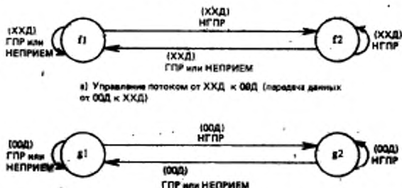
б) Управление потоком от ООД к ХХД (передача данных от ХХД к ООД)
