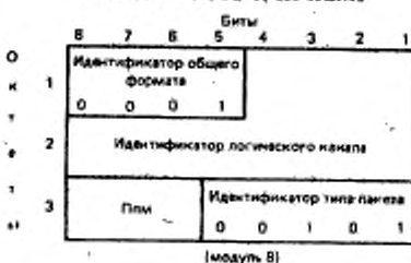
Формат пакета НЕГОТОВНОСТЬ К ПРИЕМУ
