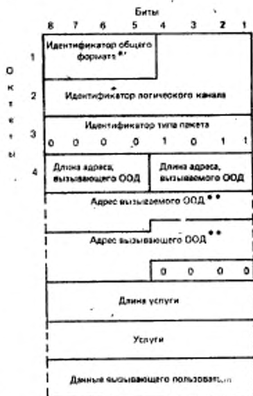
Формат пакета ЗАПРОС ВЫЗОВА и ВХОДЯЩИЙ ВЫЗОВ
