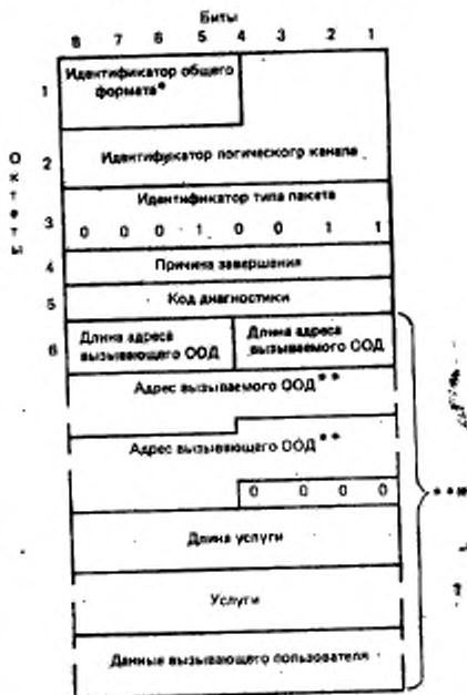
Формат пакета ЗАПРОС ЗАВЕРШЕНИЯ и ИНДИКАЦИЯ ЗАВЕРШЕНИЯ
