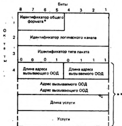
Формат пакета ПОДТВЕРЖДЕНИЕ ЗАВЕРШЕНИЯ
