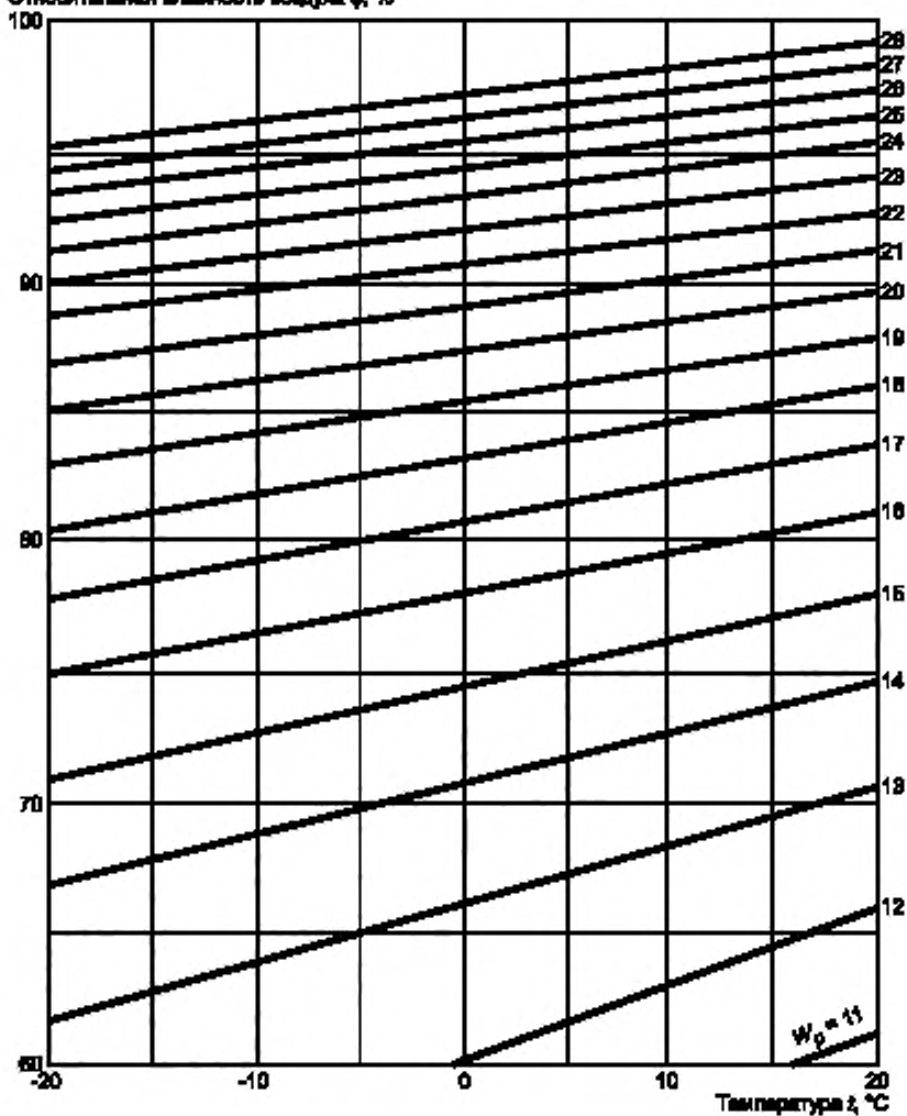
Рисунок А.19 — Диаграмма равновесной влажности
