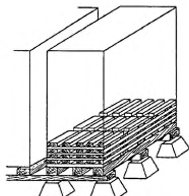
Рисунок А.18 — Укладывание заготовок
