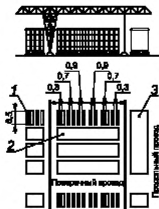
Рисунок А.4 — Планировка групп штабелей при укладывании козловым краном пиломатериалов кольцесосудистых пород, а также граба и клена
