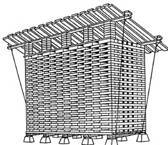
Рисунок А.17 — Составной штабель заготовок
