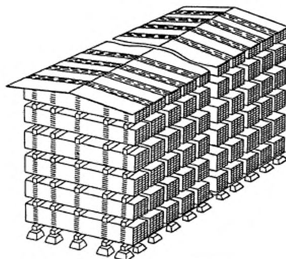
Рисунок А.14 — Пакетный штабель пиломатериалов
